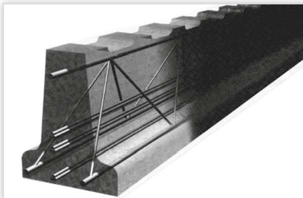
RECTOR, Belka stropowa bezpodporowa RECTOR RSE. Montaż bezpodporowy nawet do 5,8 m, idealna w przypadku renowacji (wymiany stropów), zastosowanie w stropach nad przestrzenią wentylowaną lub stropach technicznych.
